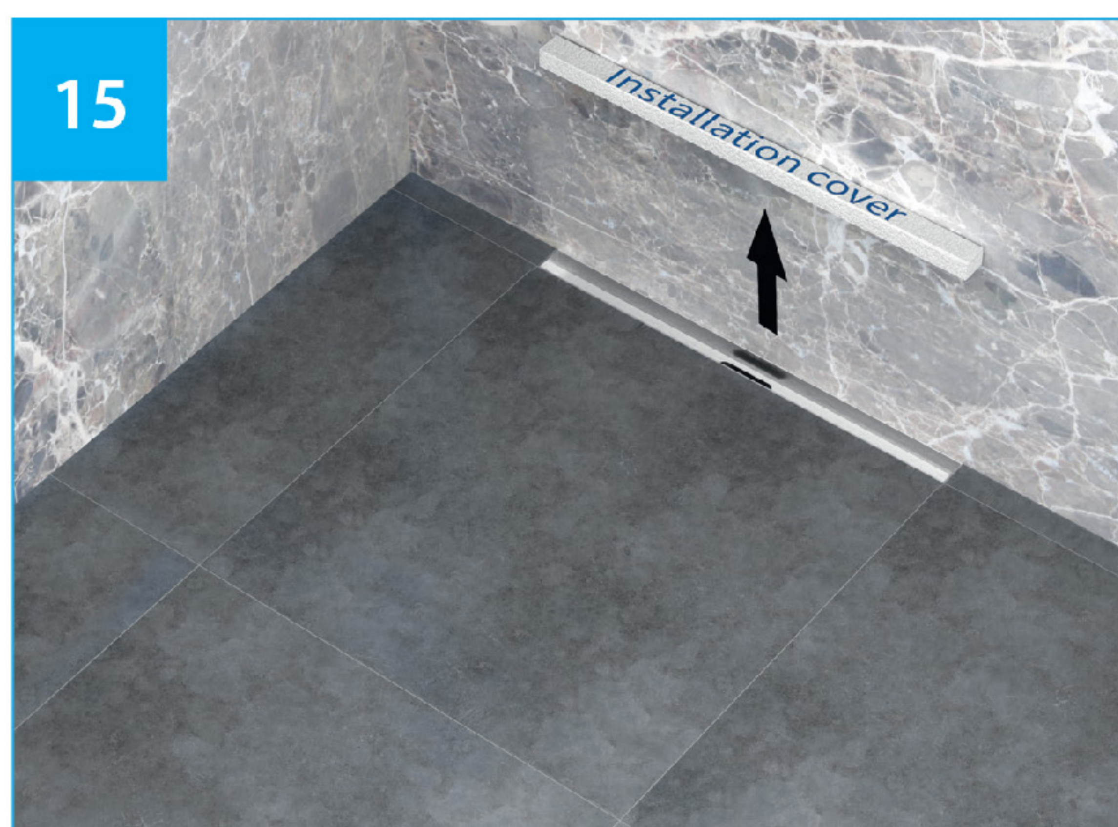
15. Wenn alles fertig und sauber gemacht wurde, kann die Montageblende entfernt werden. After finishing everything and cleaning up, the installation cover can be removed.
