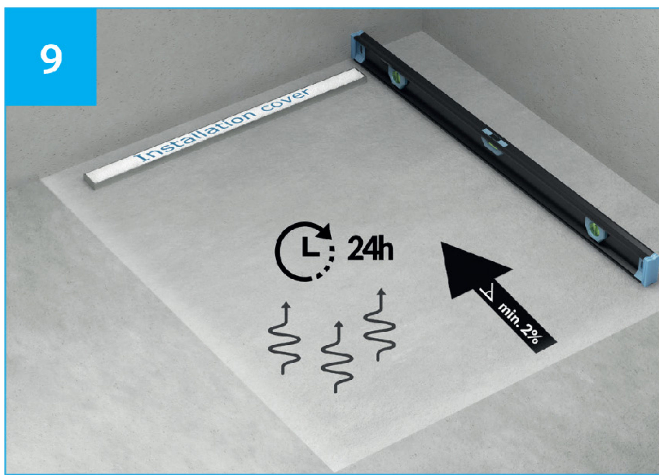
9. Arbeiten Sie ein 2%iges Gefälle in den Estrich in Richtung Duschrinne ein. Lassen Sie den Estrich 24h trocknen. Incorporate a min. 2% slope into the screed in direction of the shower drain. Let dry for 24h.
