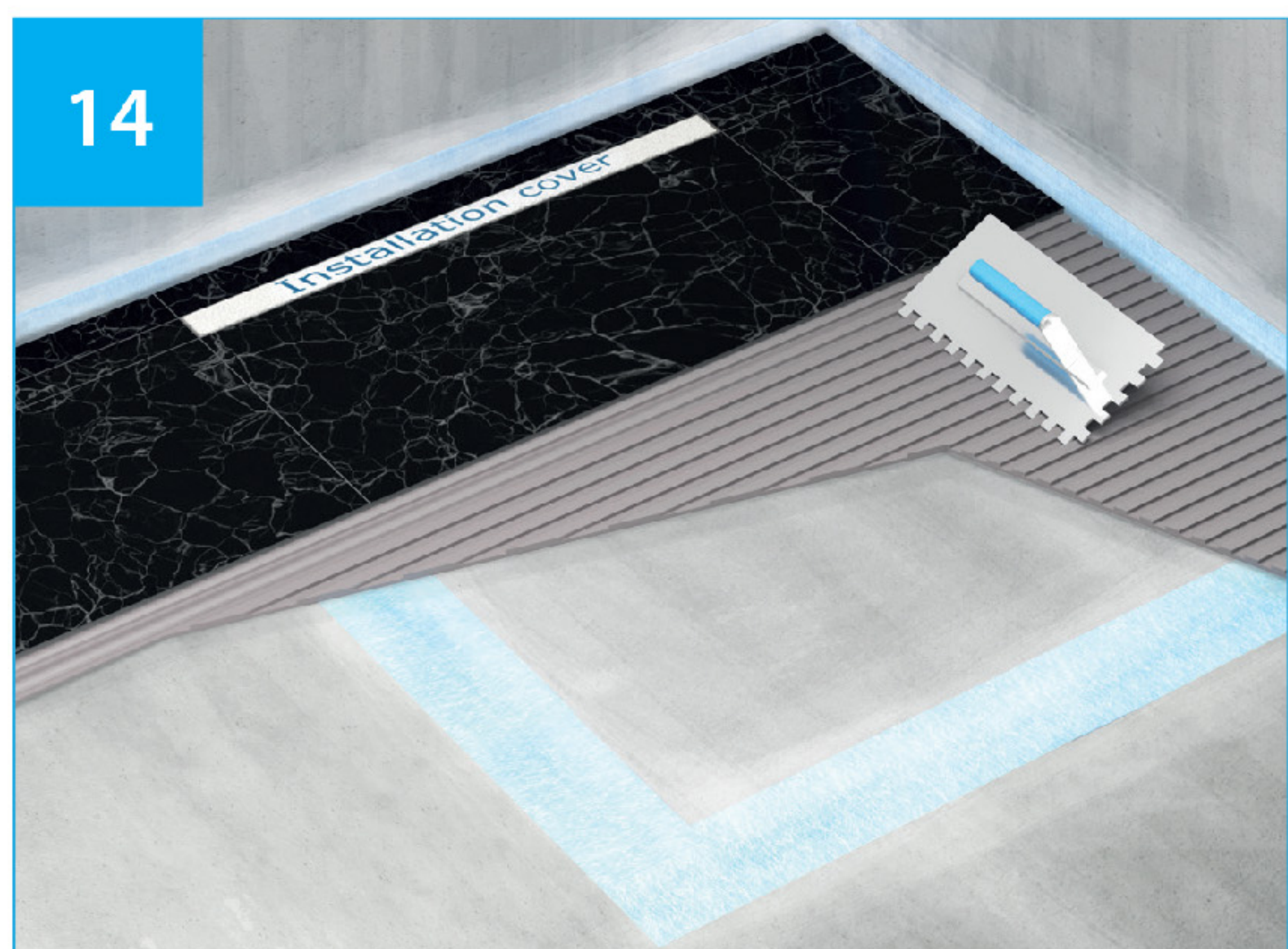
14. Verfliesen und versiegeln Sie den Duschbereich fachmännisch. Now tile and seal your shower space professionally.
