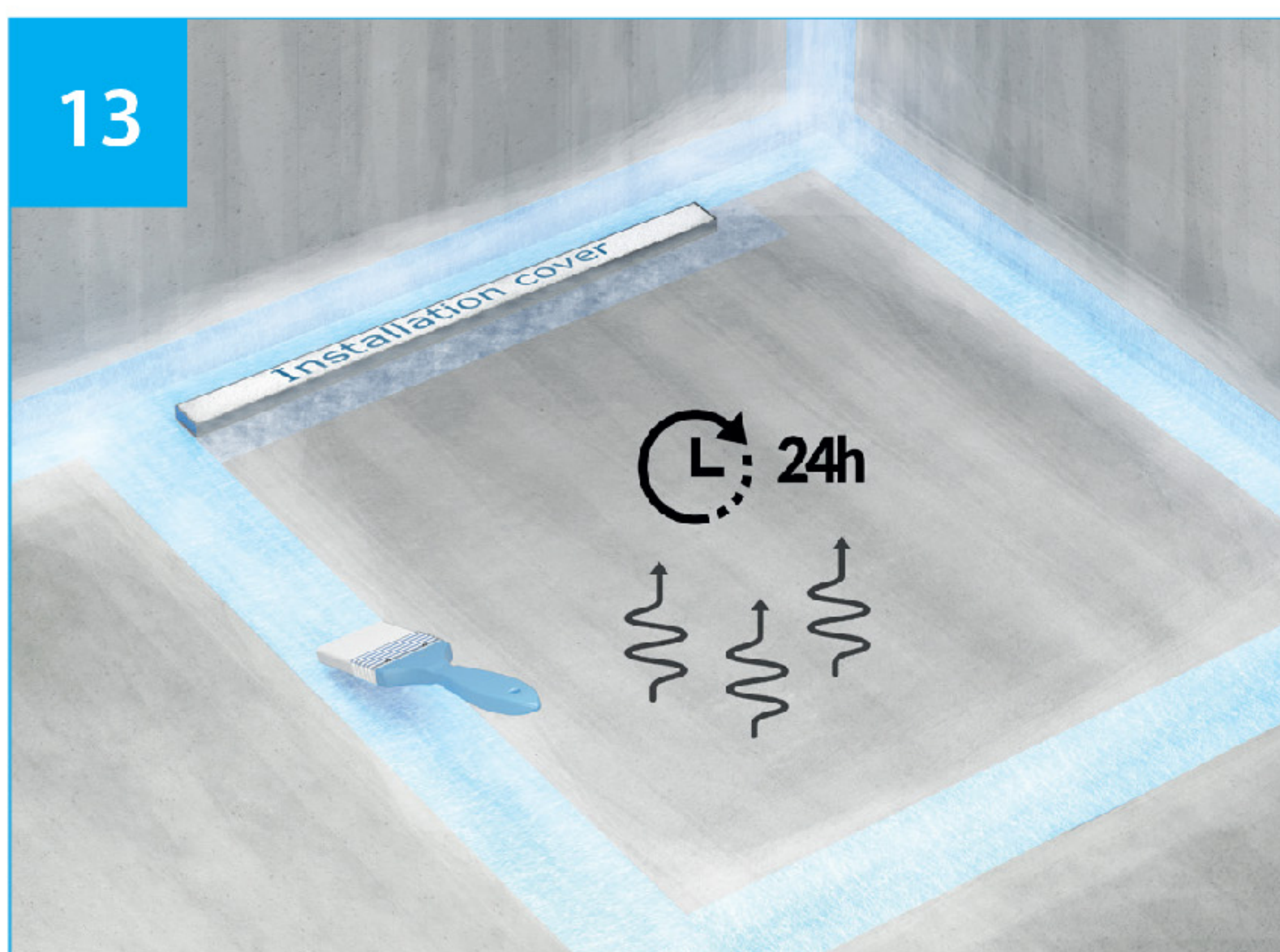
13. Lassen Sie die zweite Schicht Flüssigfolie 24 Stunden trocknen. Let the 2nd coat of liquid foil dry for 24h.
