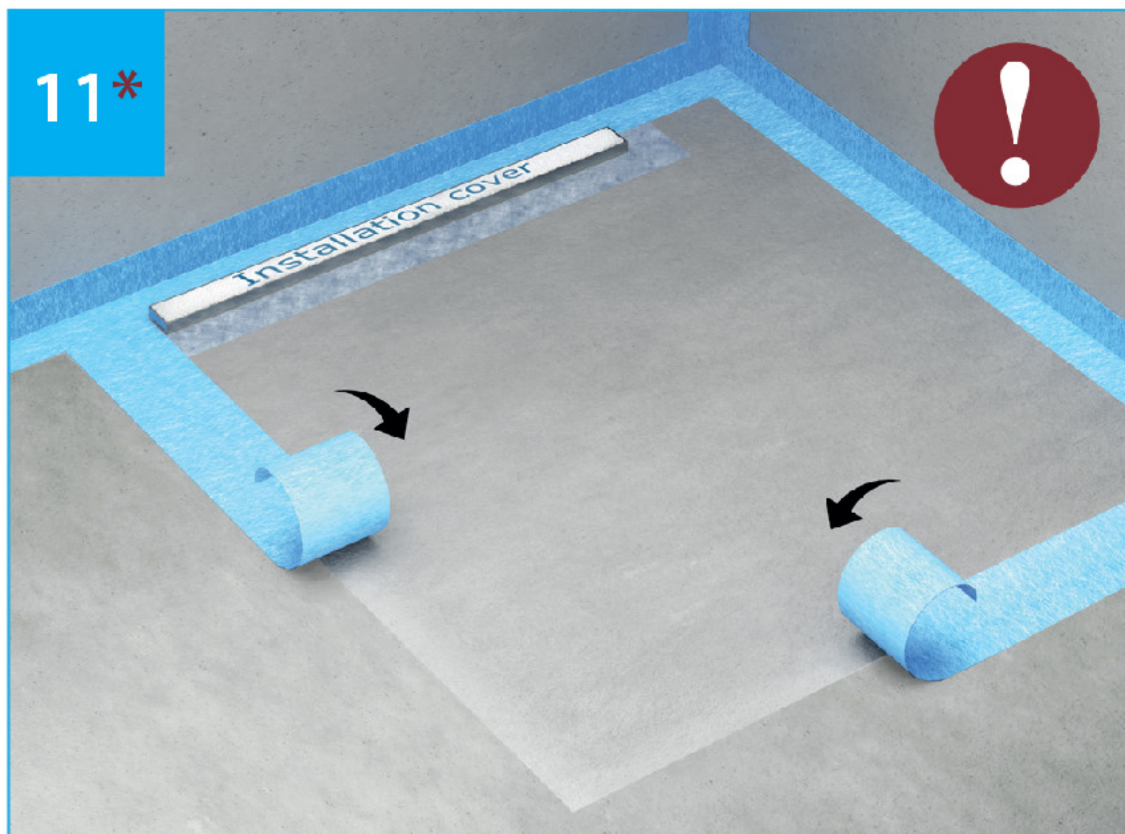
11*. Dichtband (A) + Inneneckenmanchetten (B) passend für alle Übergänge von bestehendem zu neuem Estrich zuschneiden. Cut Sealing Tape (A) + sealing corners (B) to fit all transitions from existing to new screed.
