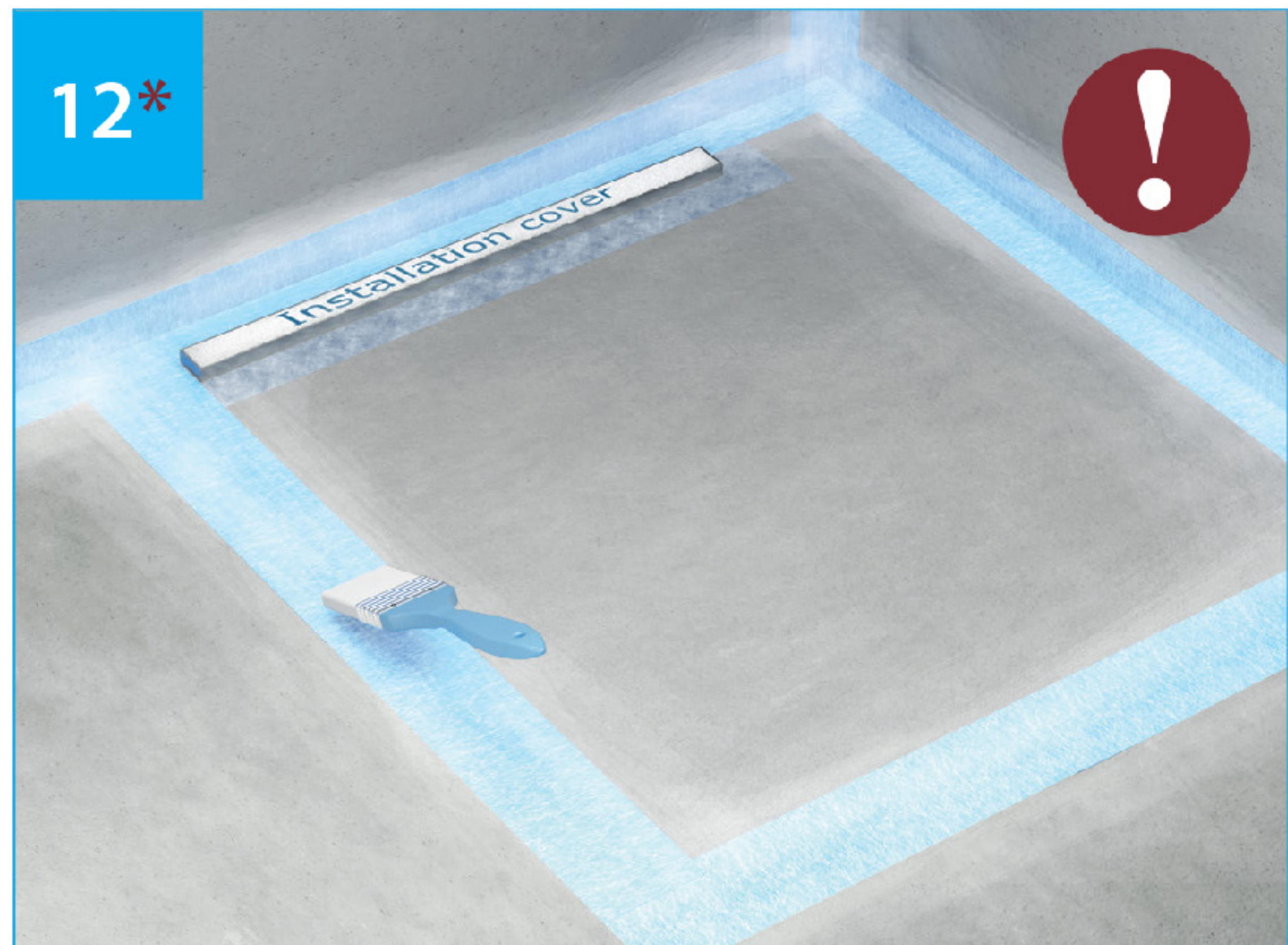
12*. Gesamten Duschbereich mit Tiefgrund streichen (24h trocknen) / A+B mit Flüssigfolie verkleben (1. Schicht, 4h) / danach weitere Schicht Flüssigfolie auftragen. Stroke whole shower area with primer (let dry for 24h) / Adhere A+B with liquid foil + whole shower area (4h let dry) / Apply 2nd coat of liquid foil.
